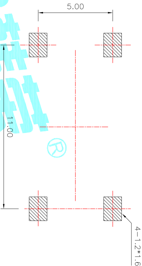
PCB Layout(Pattern side)
